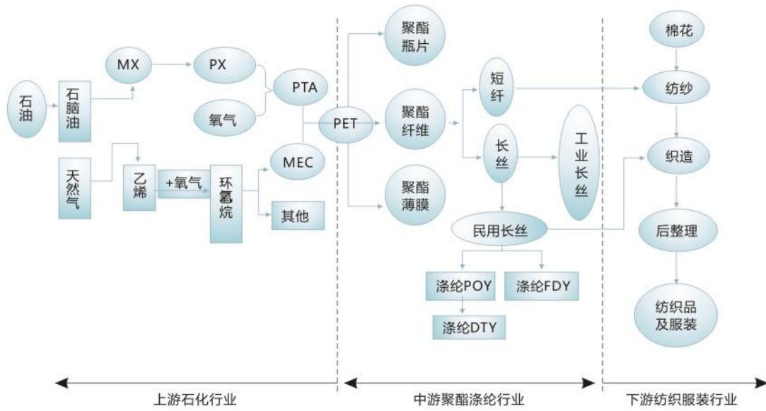
PTA产业链流程全图
